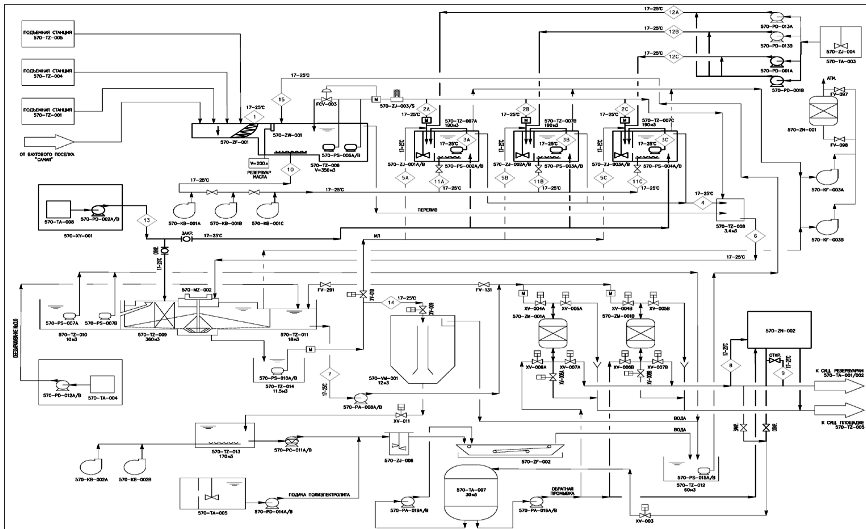
Рисунок 4.2.2 Технологическая схема УОСВ после модернизации
