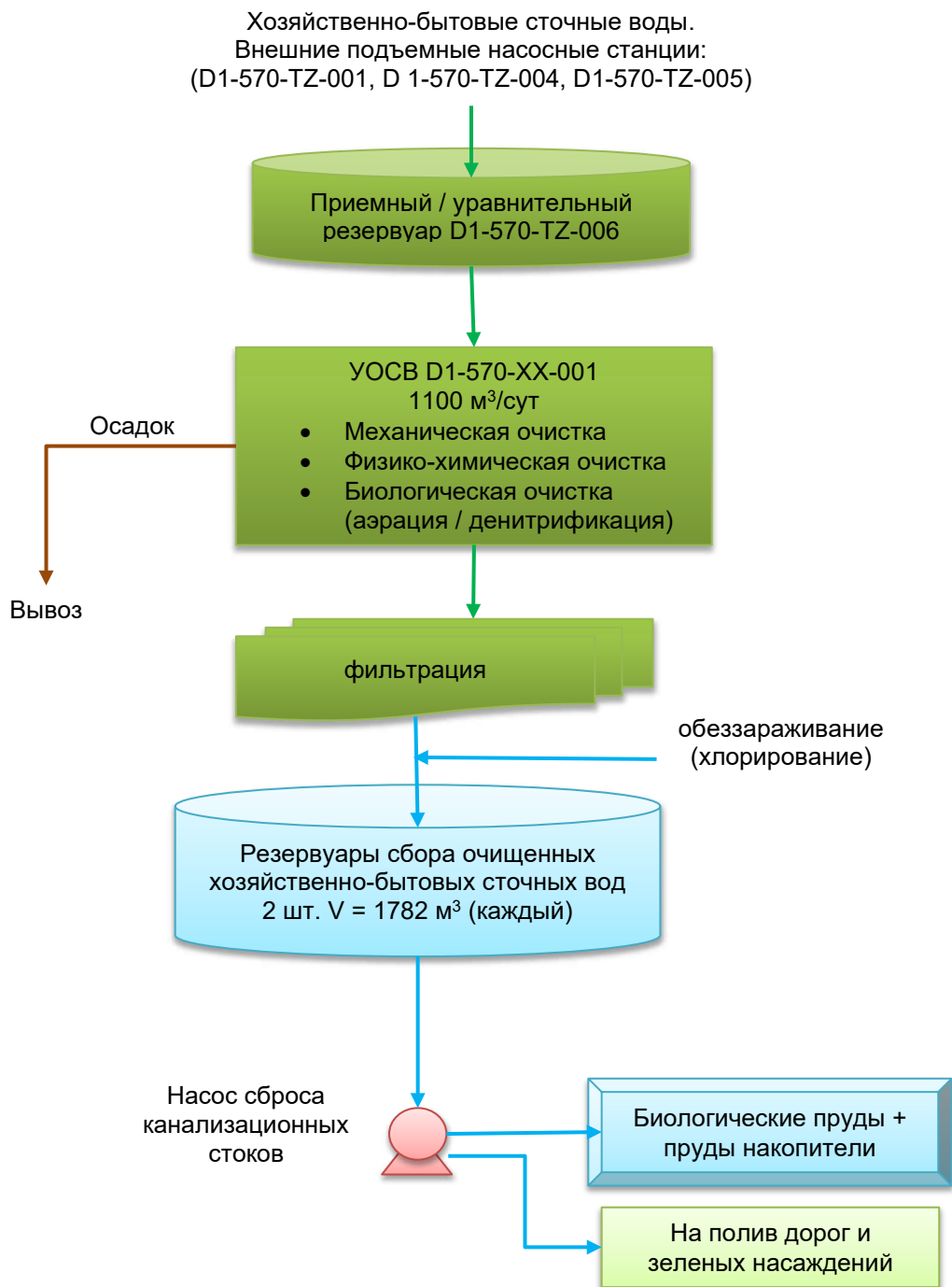
Рисунок 4.2.1 Принципиальная схема очистки хозяйственно-бытовых сточных вод
