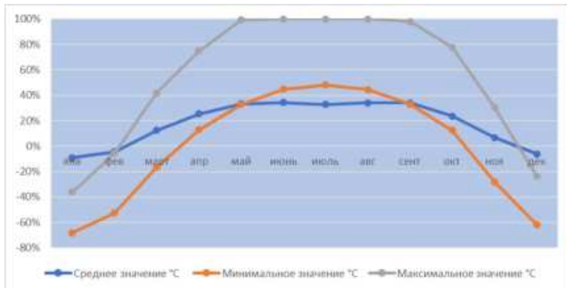
Рис.2.2.1 Годовой ход средней месячной ( T , °C), средней месячной максимальной ( T_{\max} , °C) и средней месячной минимальной ( T_{\min} , °C) температур воздуха.
