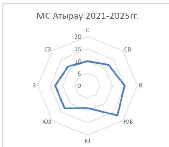
Рисунок 2.1.1 Роза ветров по м/с Атырау
