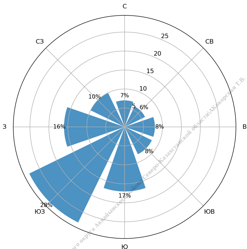
Рисунок 3 – Роза ветров Петропавловска по 8 румбам
