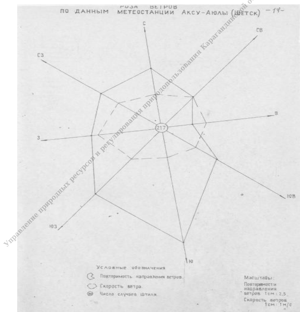
Рисунок 1. Роза ветров
