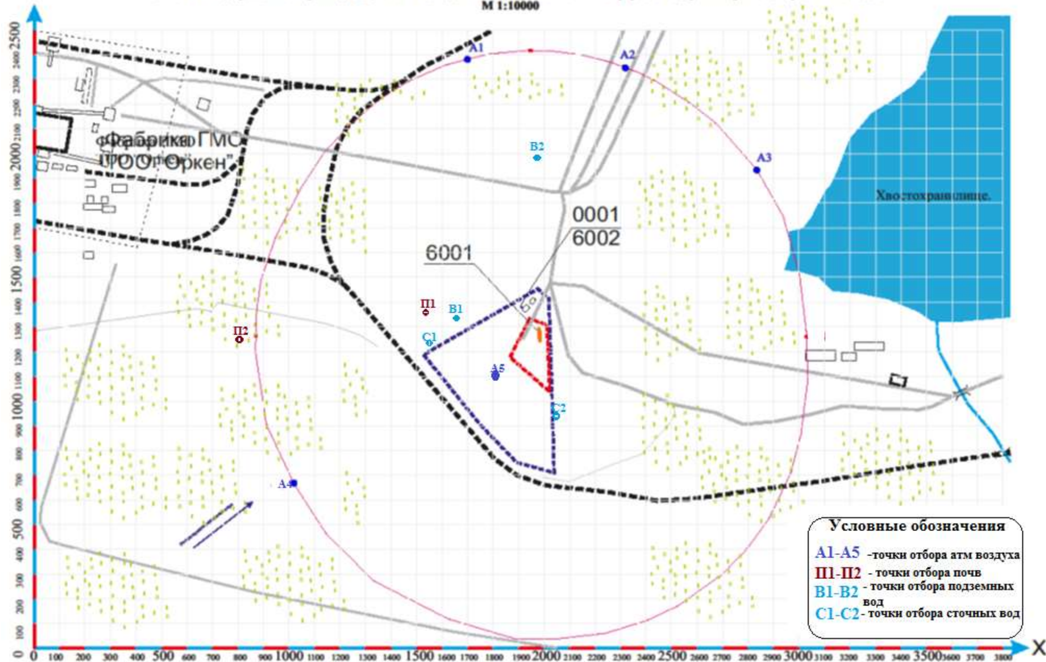
Ситуационная карта схема района размещения Полигона ТБО, с указанием границ СЗЗ, точек наблюдения за загрязнением атмосферного воздуха на границе нормативной СЗЗ. М 1:10000
