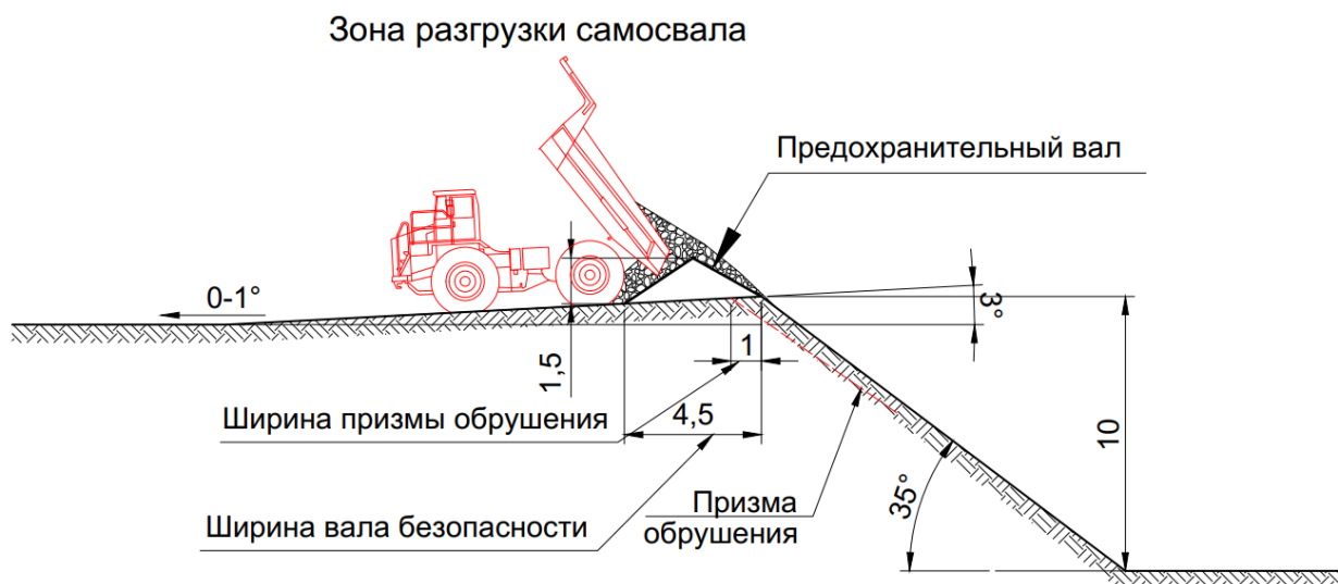
Рисунок 5.2. Схема разгрузочной площадки отвала
