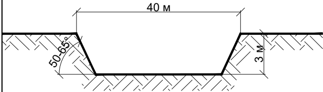
Зумпф Разрез 1-1
