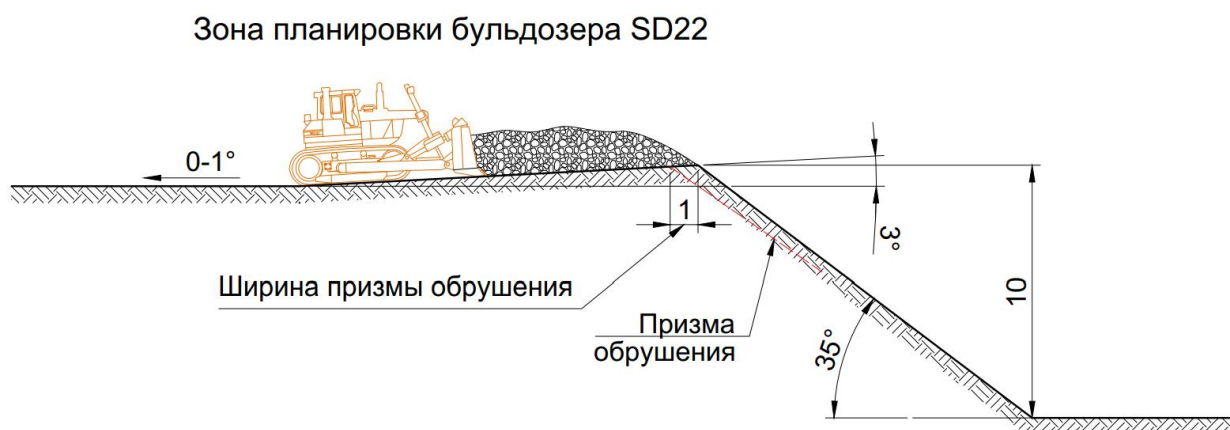
Рисунок 5.3. Формирование разгрузочной площадки отвала бульдозером
