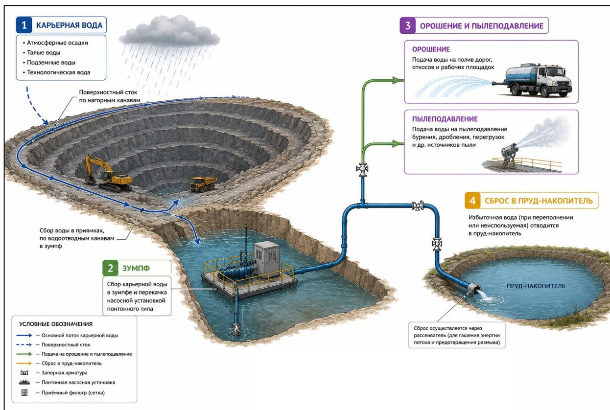
Рисунок 6.2 Схема карьерного водоотлива
