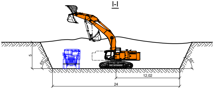
Минимальная ширина рабочей площадки
