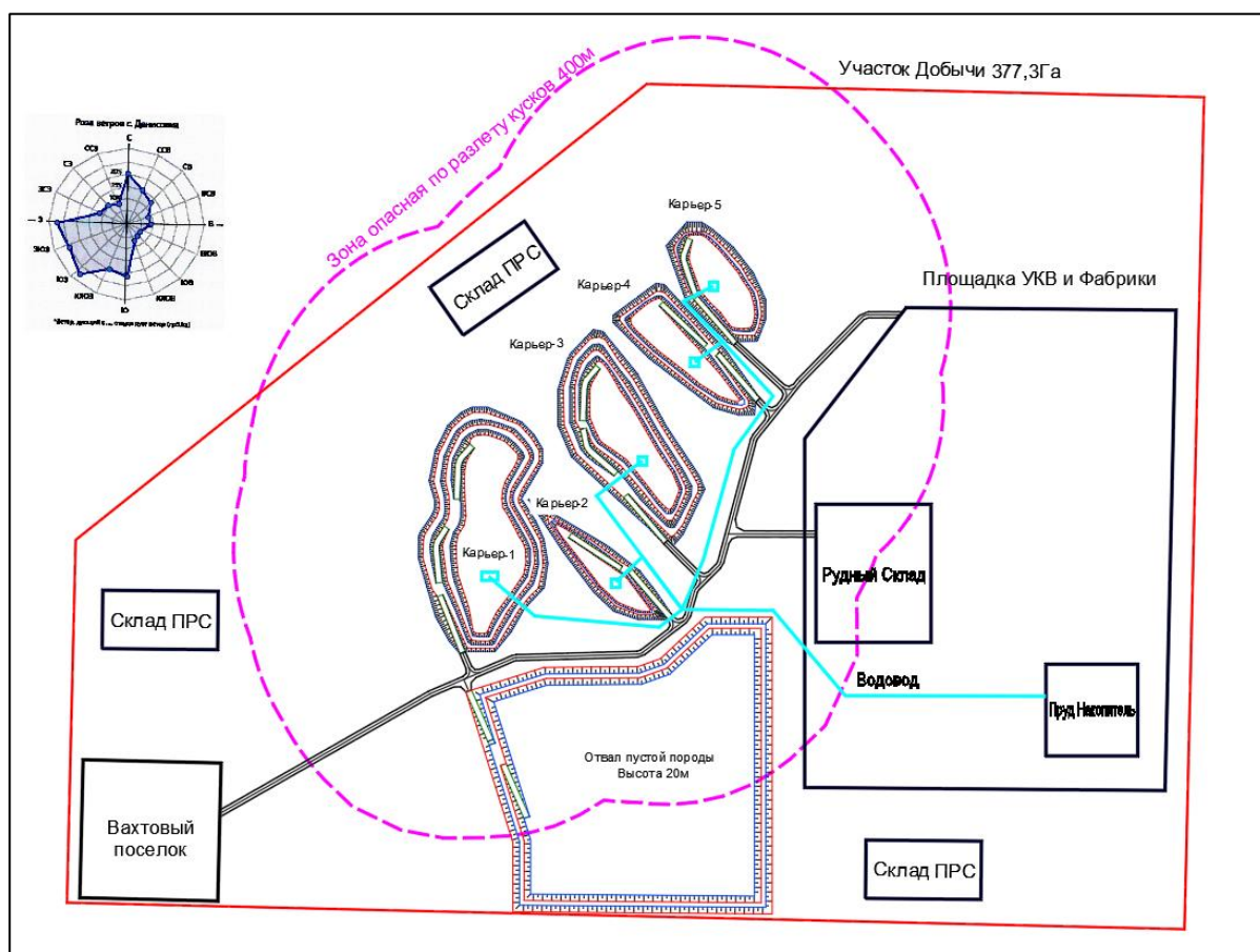
Рисунок 6.3 Схема водовода
