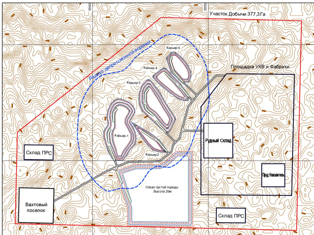
Рисунок 6.1 - Радиус депрессионной воронки
