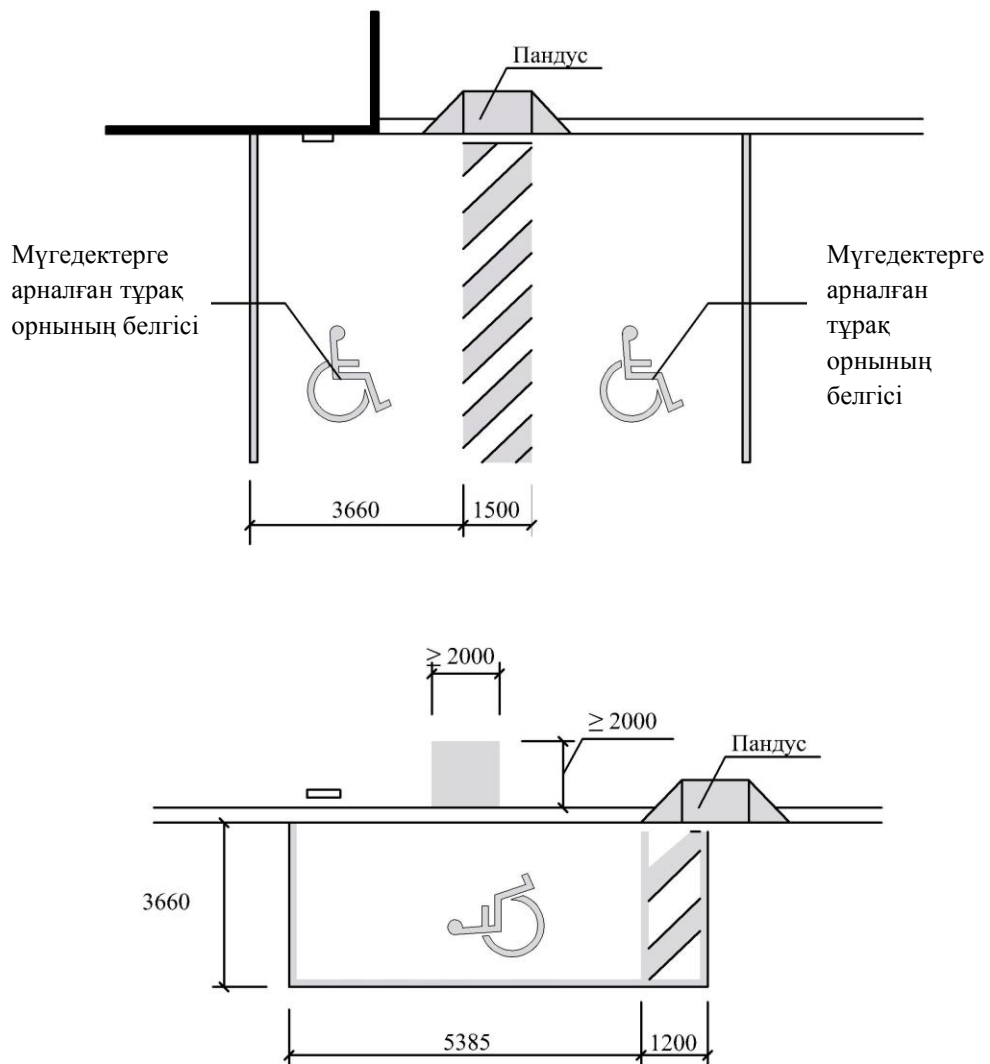
Г.1-сурет. Халықтың қимылы шектеулі топтарына арналған автотұрақ орындары
