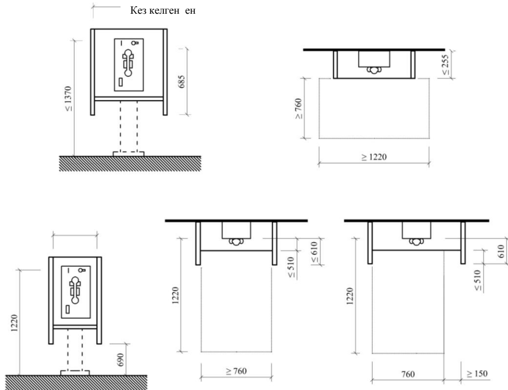
Е.1-сурет. Қоғамдық телефондар габариттері
