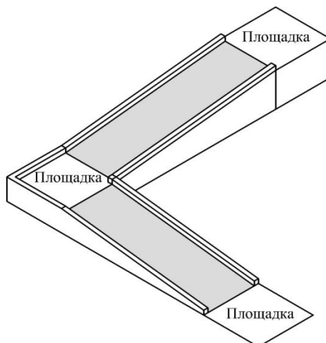
Рисунок 5 – Оформление пандусов
