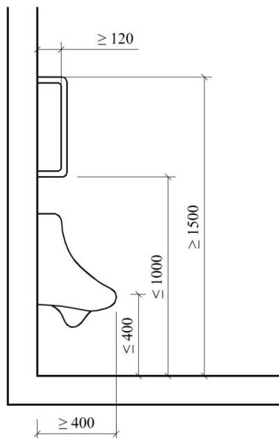
Рисунок М.3 – Ориентировочные параметры писуаров
